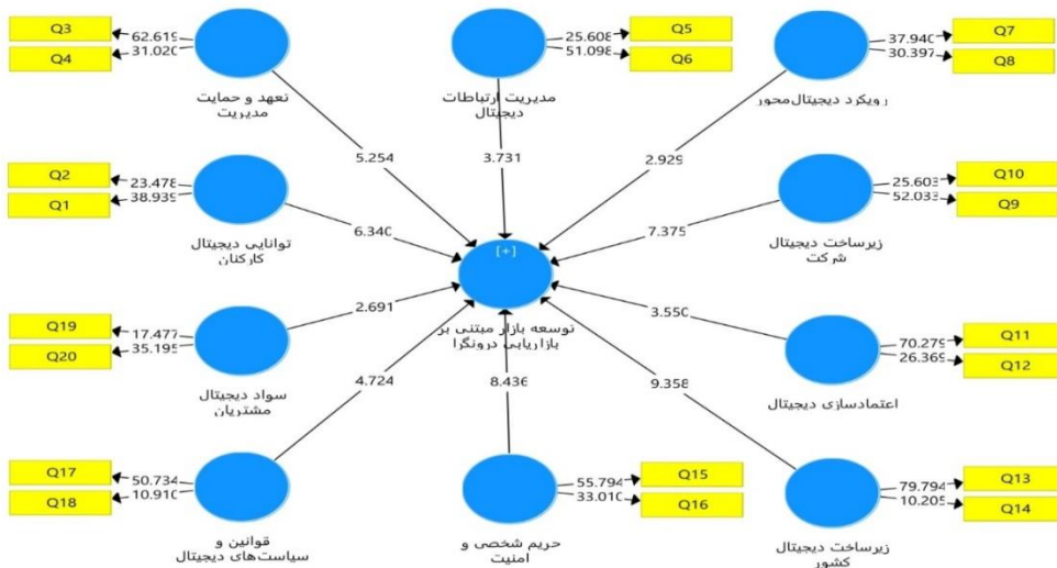
شکل ۲- ضرایب آماره t-value
